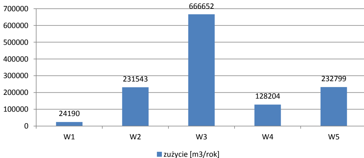
Rysunek 10. Roczna dystrybucja gazu w odniesieniu do grup taryfowych - rok 2010
